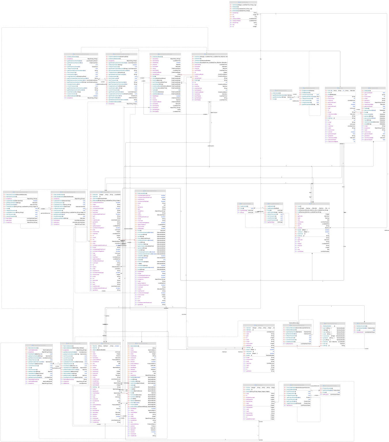
Databank schema
